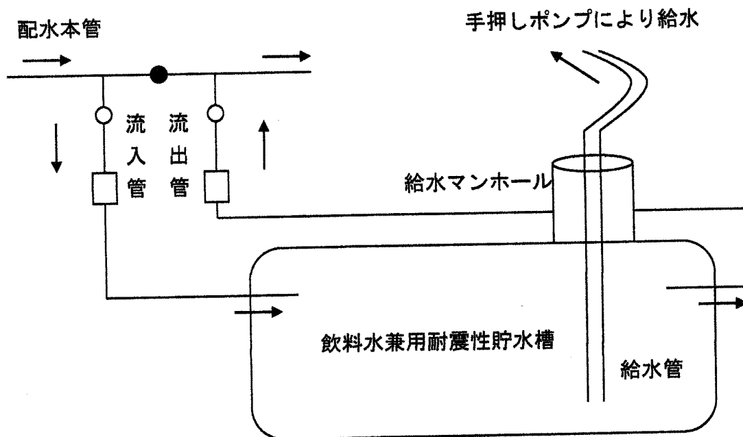
飲料水兼用耐震性貯水槽標準図
